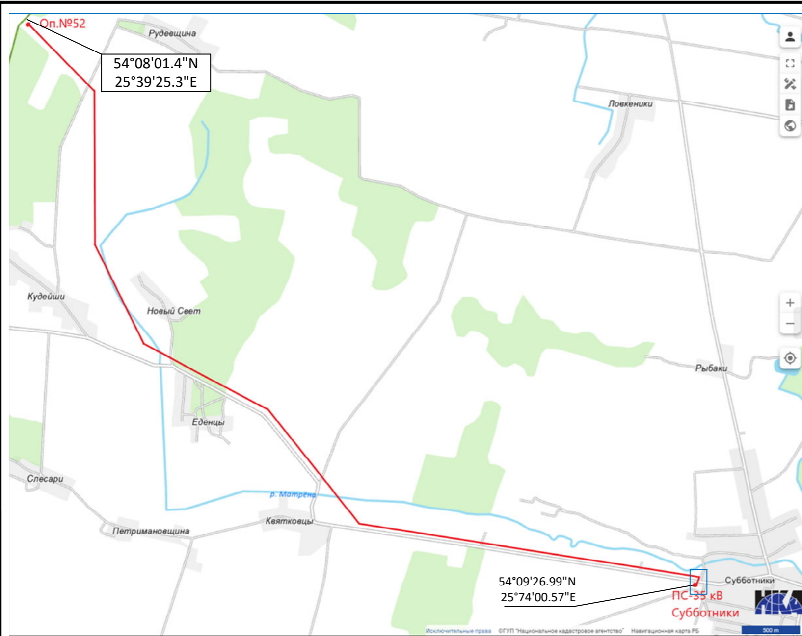
ПС 35 кВ «Субботники» с подъездной автодорогой
